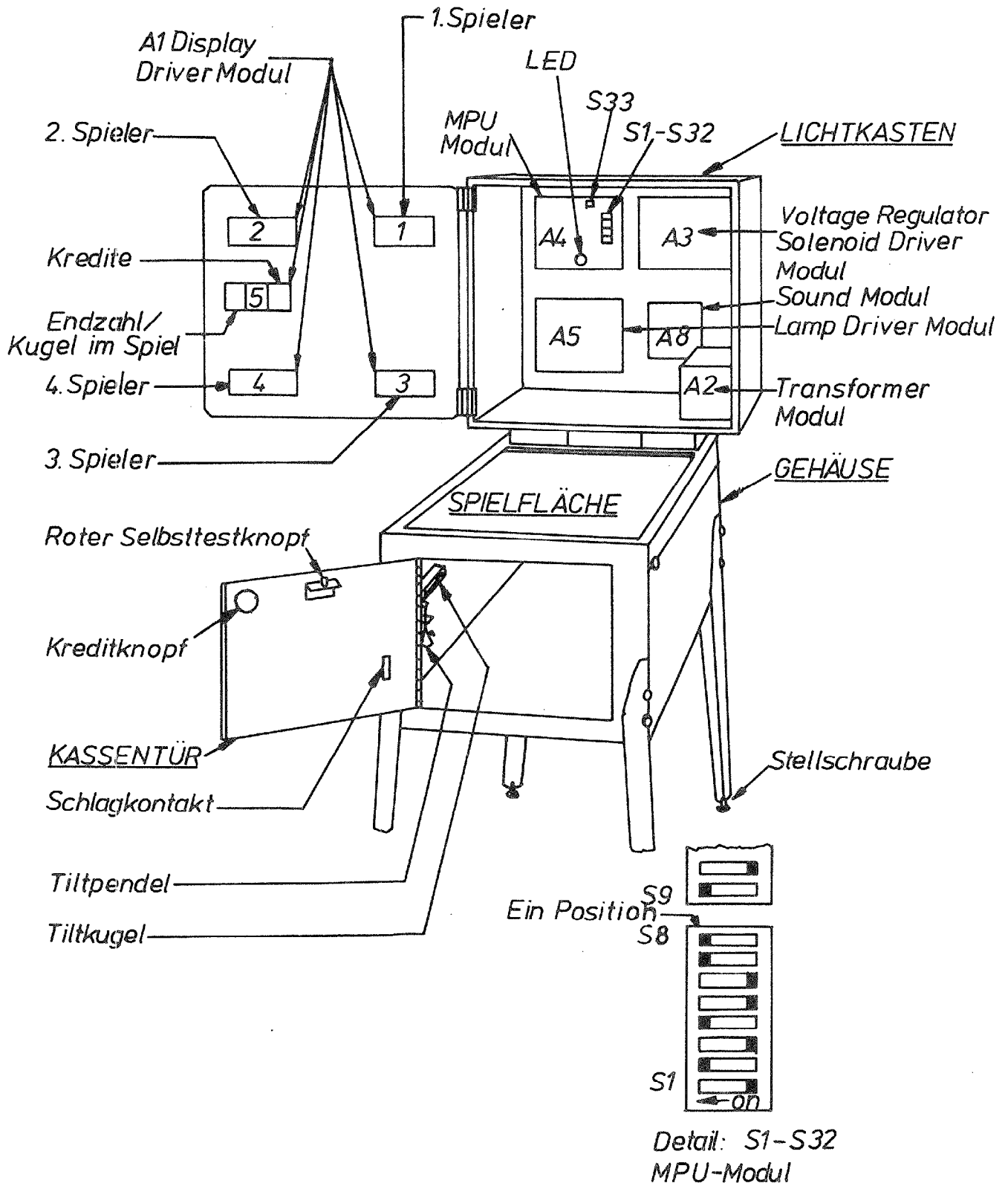
Abb. 2 Modullegeplan
