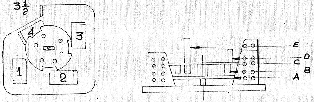
Posición de los contactos en el repetidor
