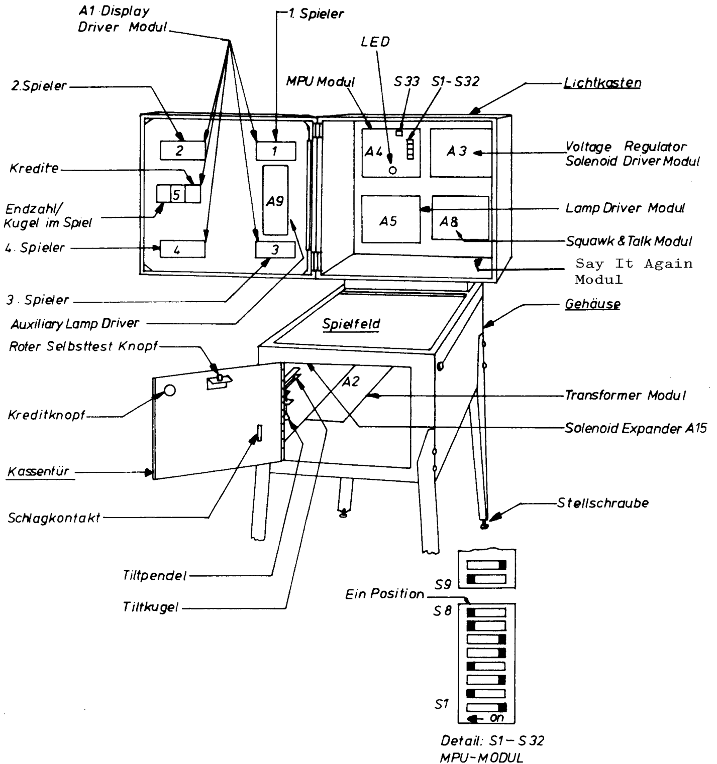
Abb. 2 Modullageplan
