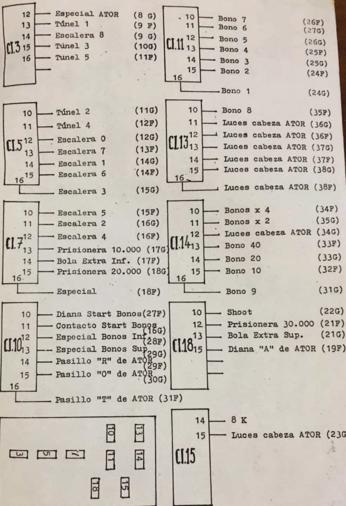
CIRCUITO DE LUCES DE LA PLACA DE JUEGO CIRCUITOS DE SALIDAS DE LUCES DEL TABLERO DE JUEGO
